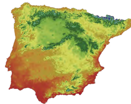
Temperatura en °C sobre superficie horizontal en primavera-verano.
