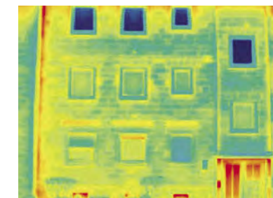
Imagen termográfica, después de la rehabilitación con Termoklinker. La pared externa está aislada térmicamente.
